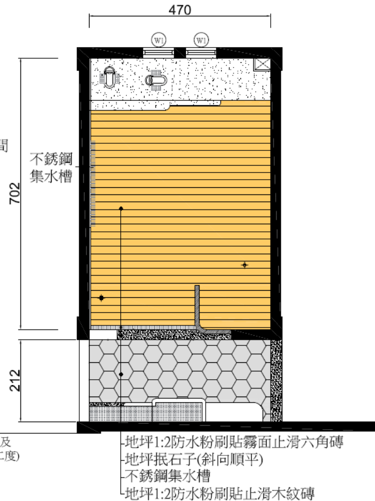
二、四樓廁所地坪整修平面圖 S:1/100
