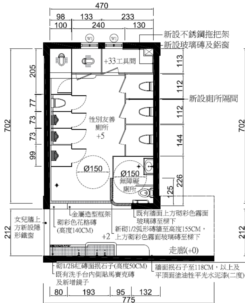
二、四樓廁所整修平面圖 S:1/100
