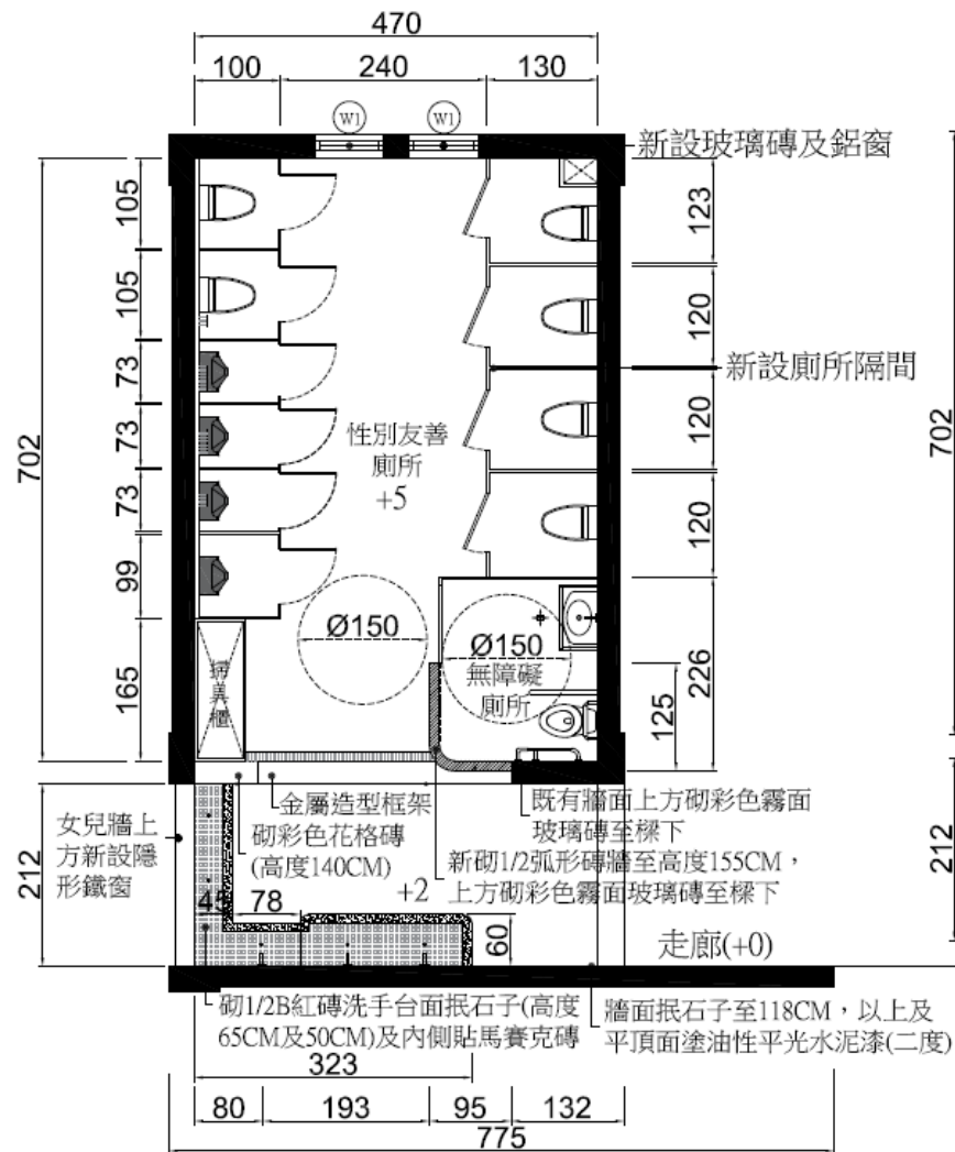
三樓廁所整修平面圖 S:1/100
