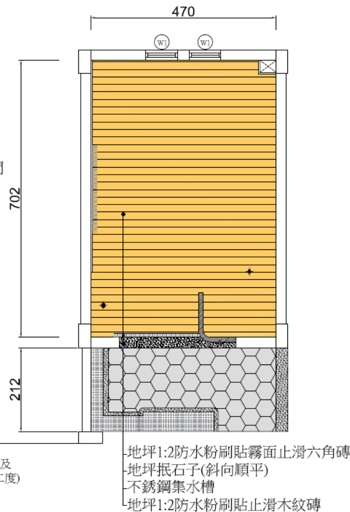
三樓廁所地坪整修平面圖 S:1/100
