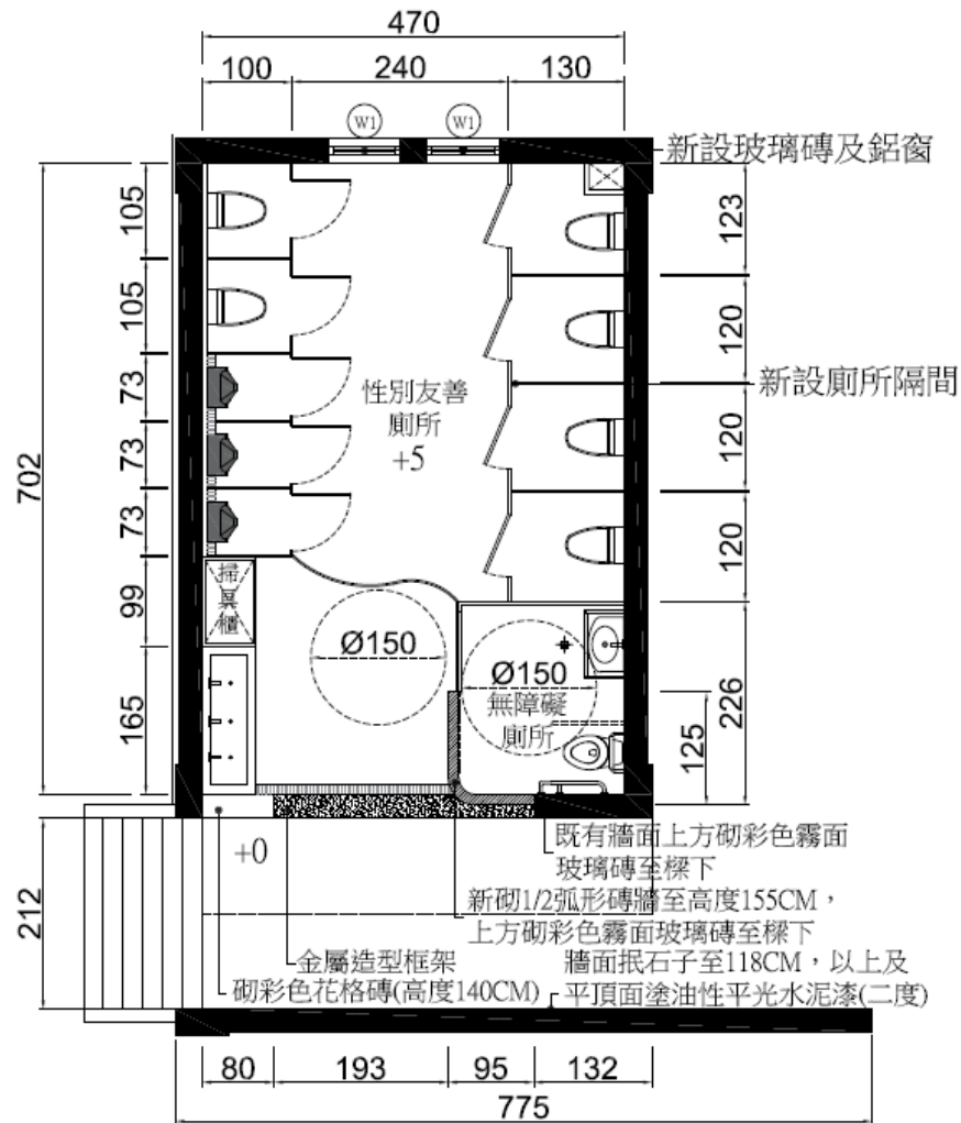
一樓廁所整修平面圖 S:1/100
